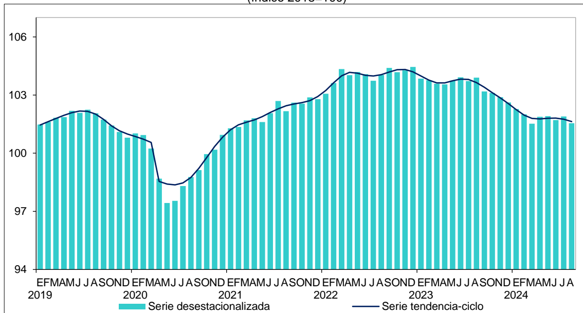
Gráfica 1 SERIE DESESTACIONALIZADA Y DE TENDENCIA-CICLO DEL PERSONAL OCUPADO TOTAL a agosto de 2024 (índice 2018=100)
