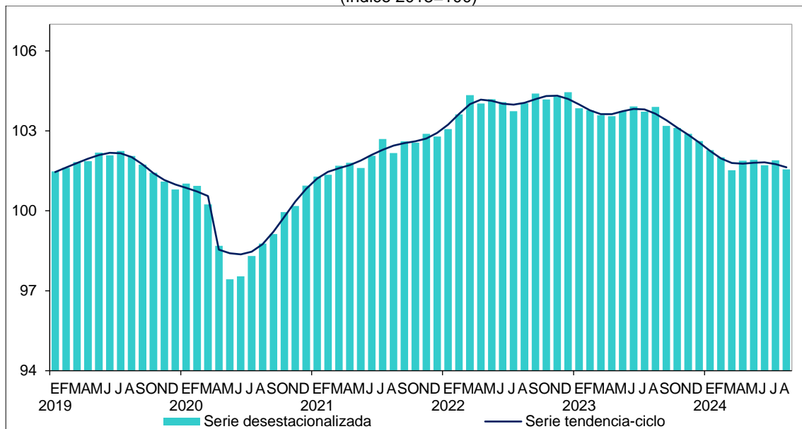
Gráfica 1 SERIE DESESTACIONALIZADA Y DE TENDENCIA-CICLO 1/ DEL PERSONAL OCUPADO TOTAL a agosto de 2024 (índice 2018=100)
