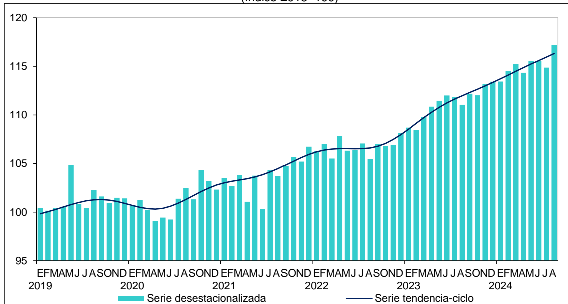
Gráfica 3 SERIE DESESTACIONALIZADA Y DE TENDENCIA-CICLO DE LAS REMUNERACIONES MEDIAS REALES PAGADAS a agosto de 2024 (índice 2018=100)
