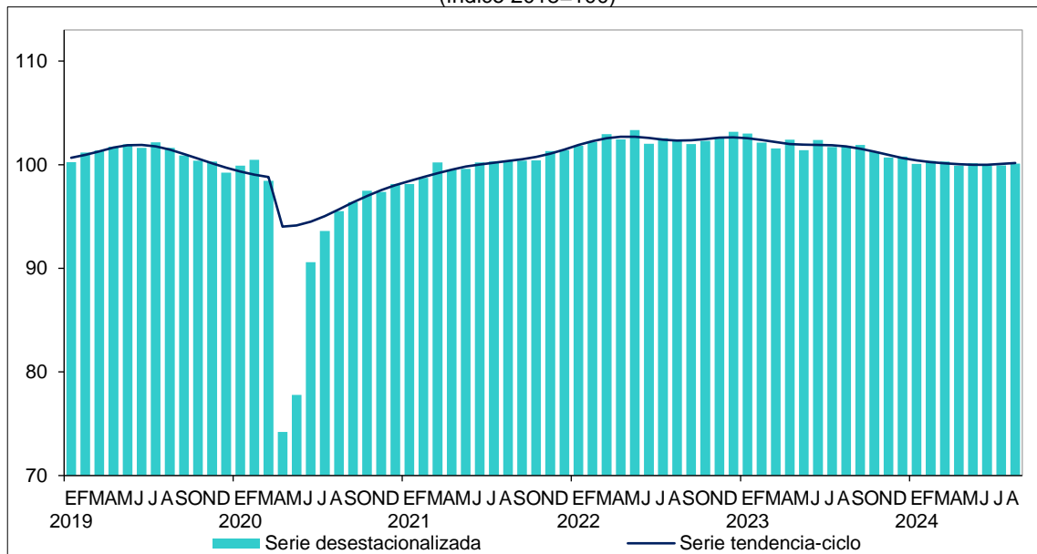
Gráfica 2 SERIE DESESTACIONALIZADA Y DE TENDENCIA-CICLO DE LAS HORAS TRABAJADAS POR EL PERSONAL OCUPADO TOTAL a agosto de 2024 (índice 2018=100)
